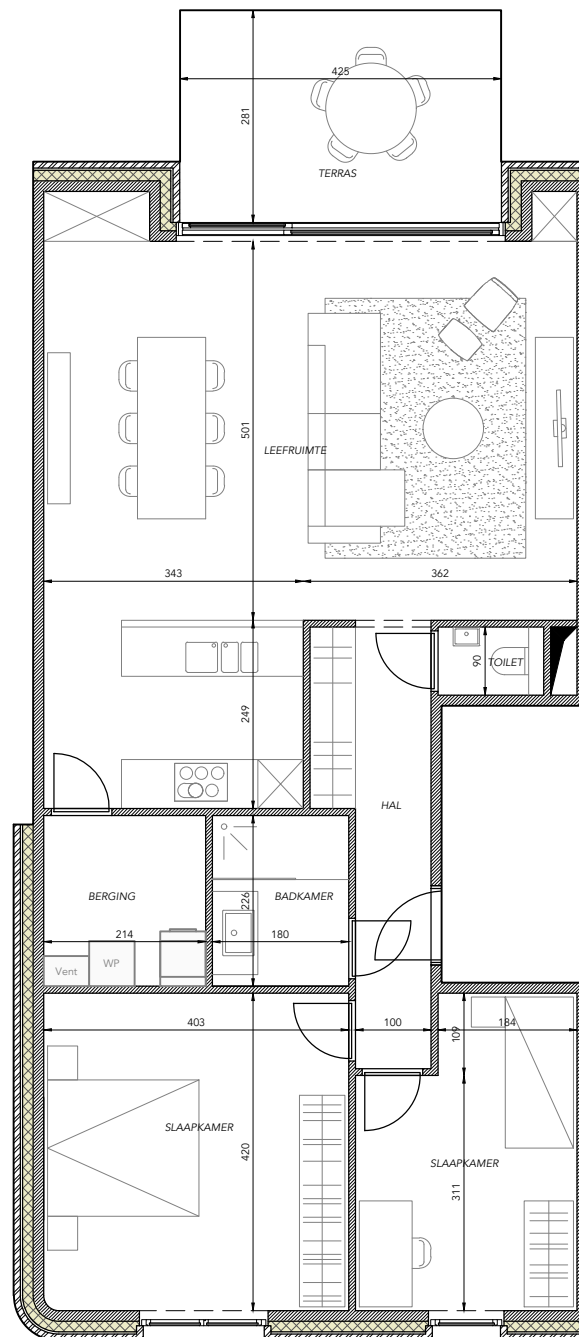
GRONDPLAN APPARTEMENT
