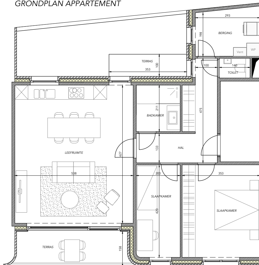
GRONDPLAN APPARTEMENT
