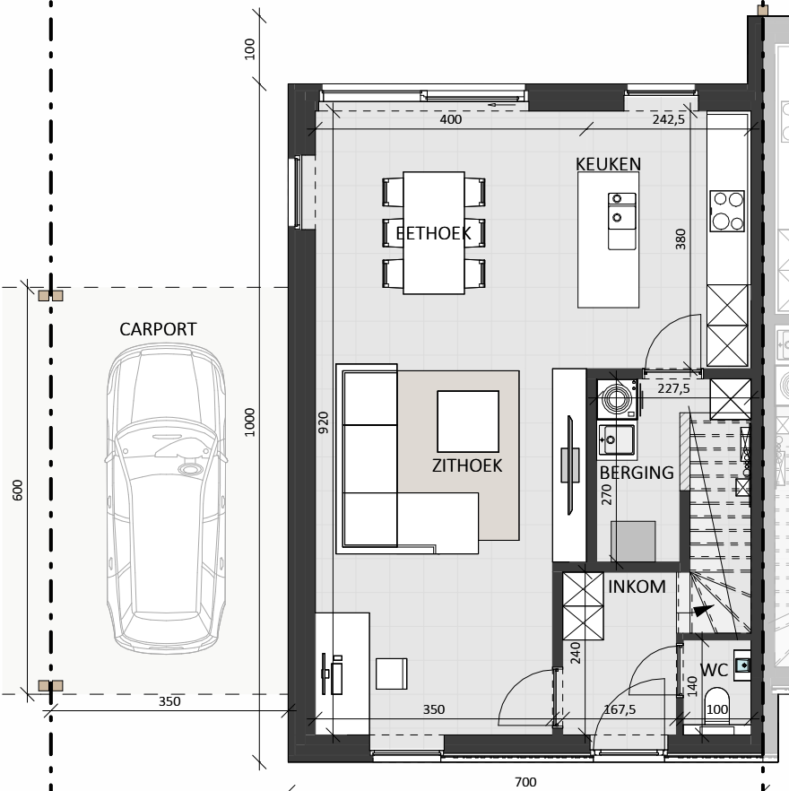
GELIJKVLOERS
