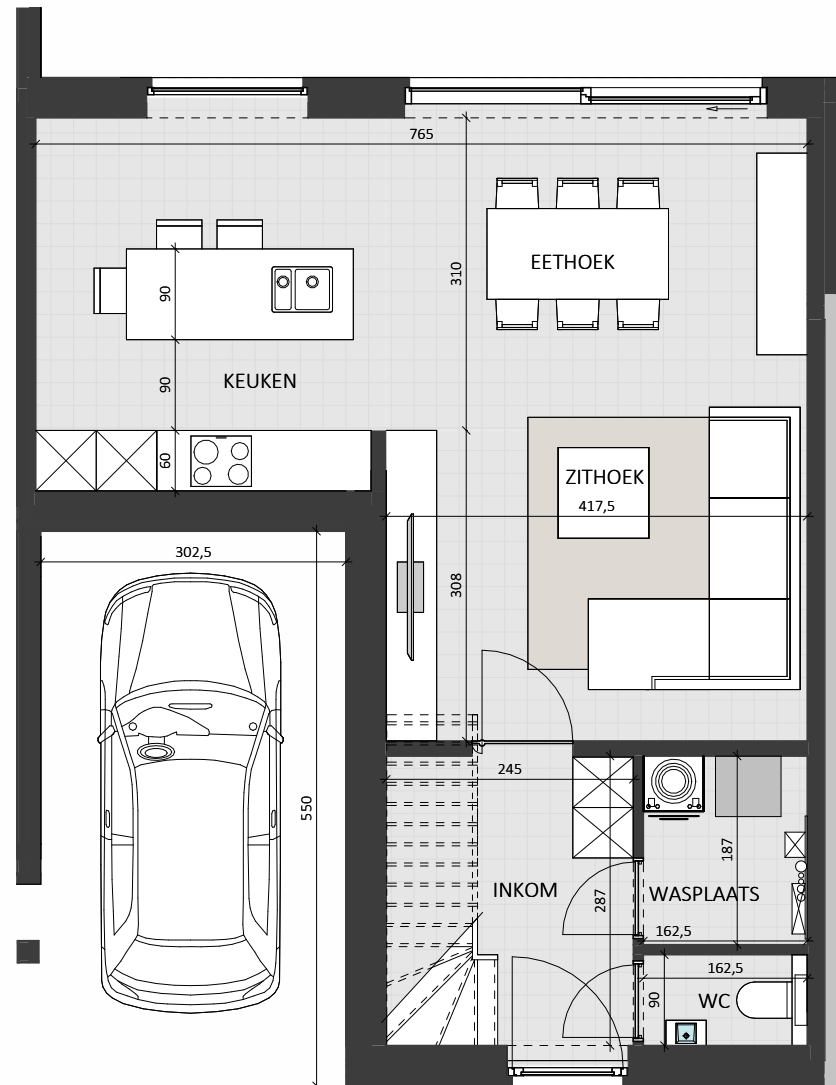
GELIJKVLOERS
