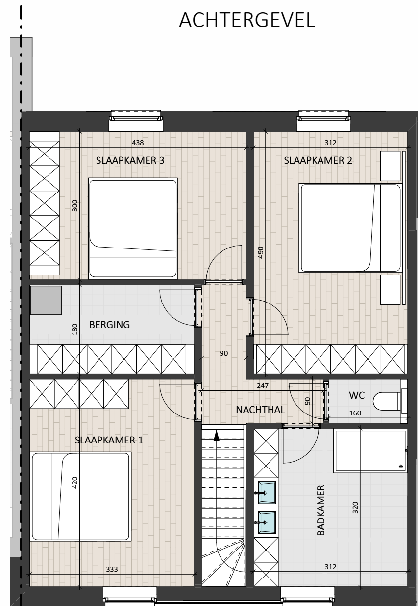
1e VERDIEPING
