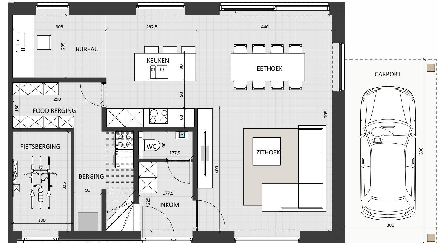
GELIJKVLOERS
